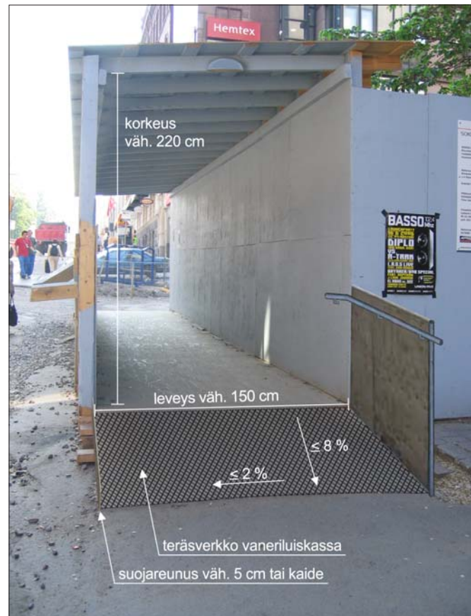
Kuva 5. Sulkuaita/sulkupuomi pitää sijoittaa täsmälleen suojatien kohtaan, jotta näkövammaisen ohjautuu oikealle reitille. Merkkien sijoituskorkeus 1,4–1,6 m.
